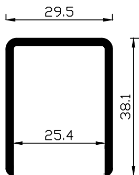
DS18 0.55 kg/m
