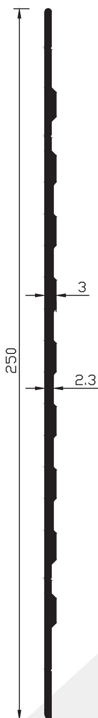
SIK5 2.10 kg/m
