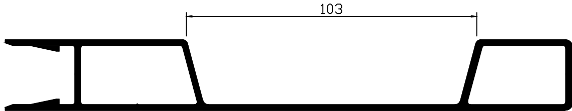
HP42A HP42M
