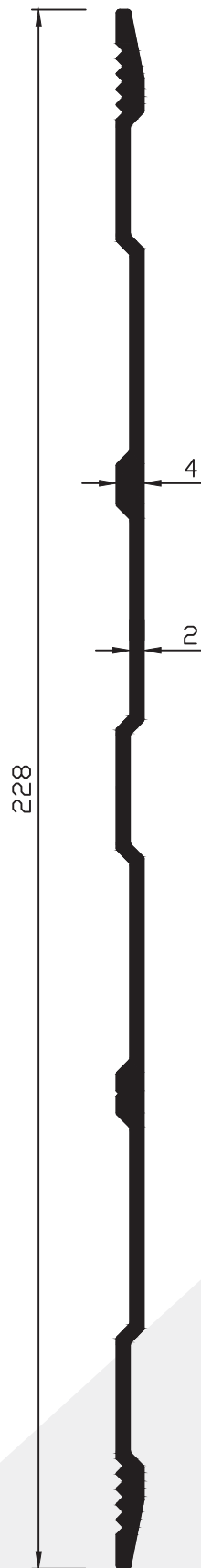
SIK1 1.58 kg/m
