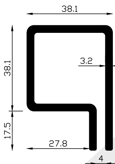
C40 0.51 kg/m
