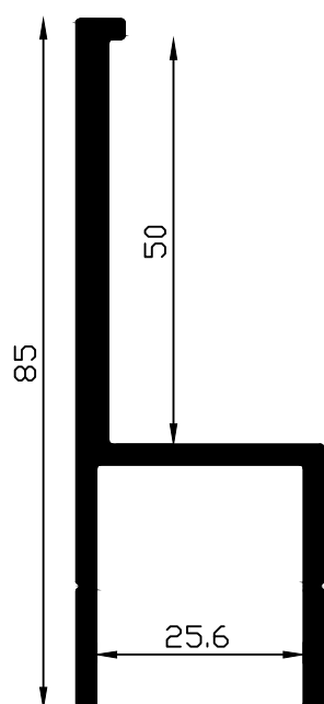
DS10 1.19 kg/m
