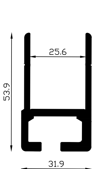
HP22 0.66 kg/m
