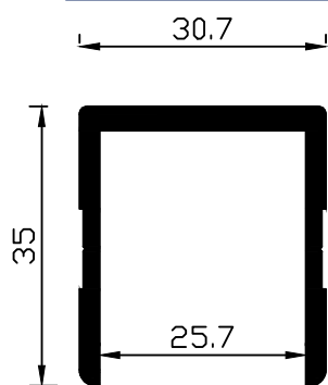
HP22 0.66 kg/m
