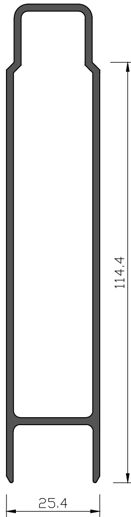
HP14 1.96 kg/m
