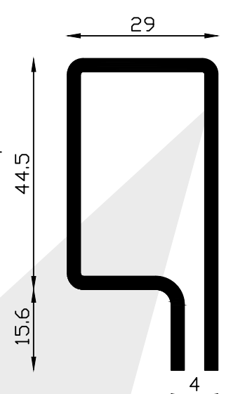
C41 0.70 kg/m
