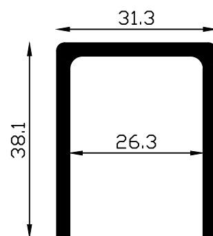
C41 0.70 kg/m
