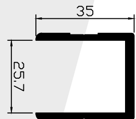
HP22A HP22M
