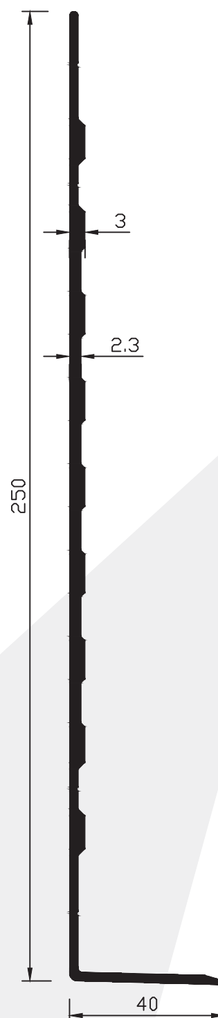
SIK4 2.32 kg/m
